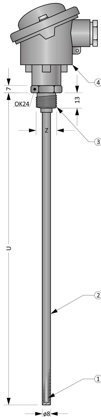
Obrázek 16N.1: MTC16N
