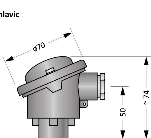
Obrázek 16N.2: Hlavice B
