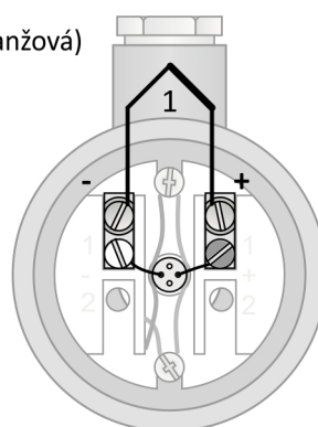
Obrázek 1L.5: zapojení jednoduchého termočlánu
