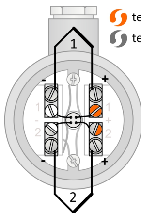
Obrázek 2C.4: zapojení dvojitého termočlánu
