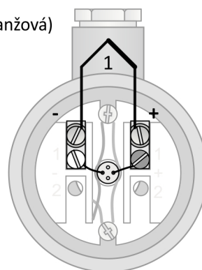
Obrázek 2C.5: zapojení jednoduchého termočlánu
