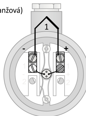
Obrázek 2L.5: zapojení jednoduchého termočlánu
