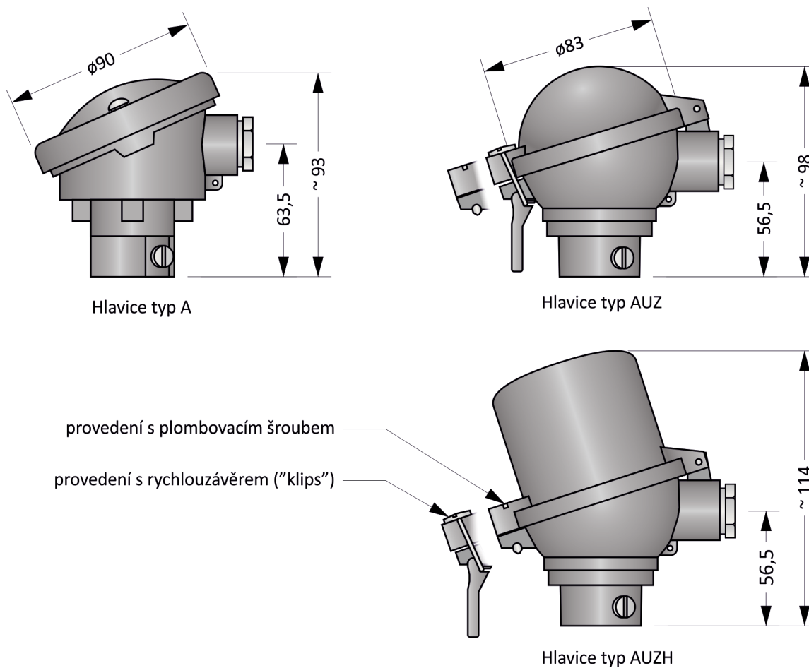
Obrázek 4.2: Typy hlavic
