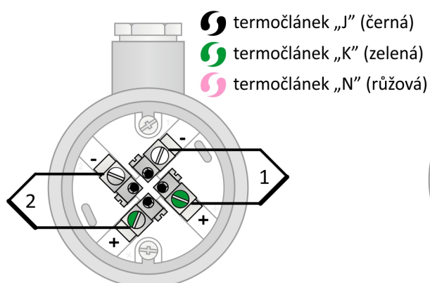
Obrázek 8.3: zapojení dvojitého termočlánu
