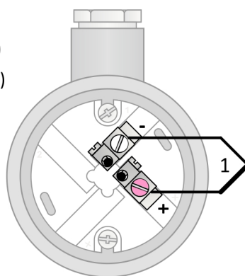
Obrázek 8.4: zapojení jednoduchého termočlánu
