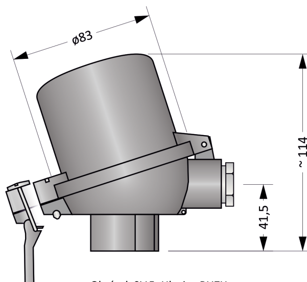
Obrázek 9V.5: Hlavice BUZH
