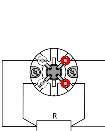
Obrázek 15.3: RTD v čtyřvodičovém zapojení
