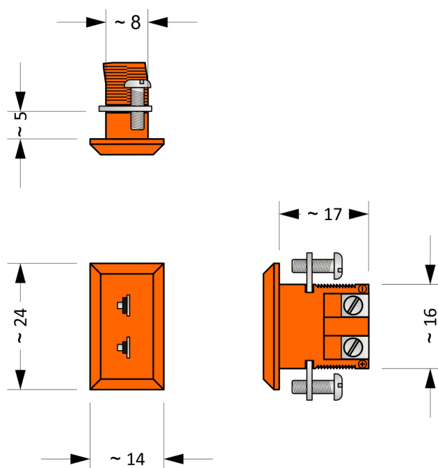
Obrázek MK.PM.1: zásuvka MTCK-PMIFB-J
