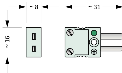
Obrázek MK.CM.1: konektor MTCK-CMM-K
