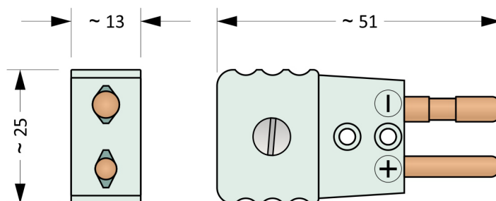
Obrázek MK.LS.1: konektor MTCK-LSM-CU
