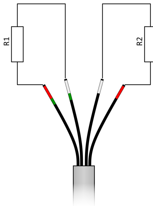
Obrázek 10.7: 2 x RTD v dvouodičovém zapojení
