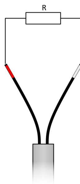
Obrázek 10.5: RTD v dvouodičovém zapojení
